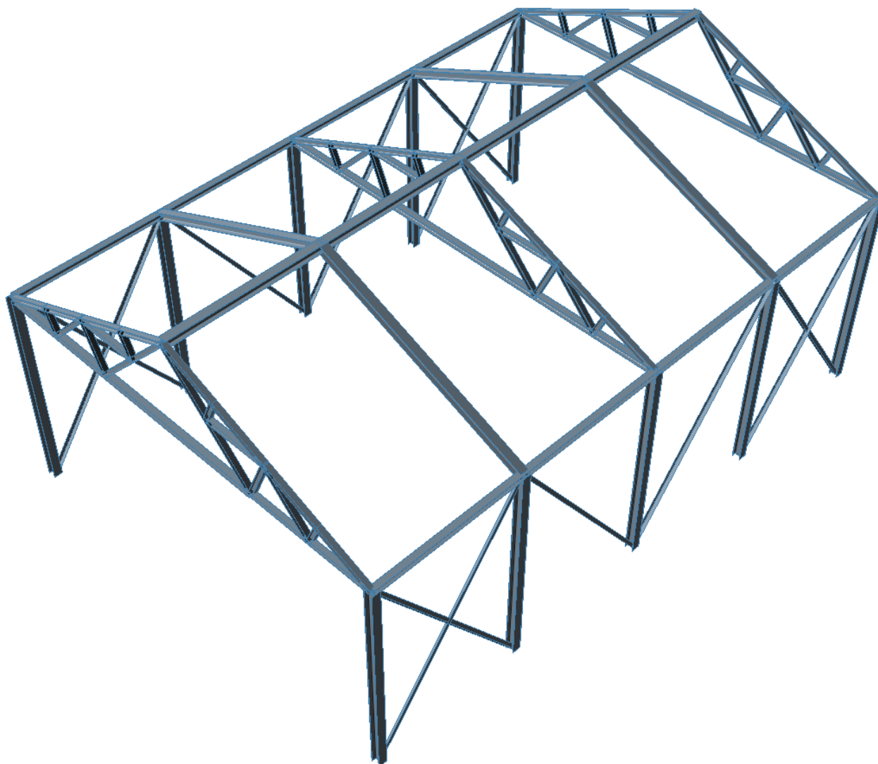
immagine del modello di calcolo del capannone in acciaio
